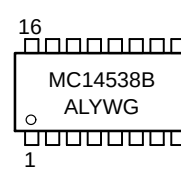
SOEIAJ-16
