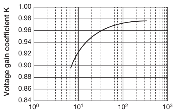
Fig. 1 R_g (kΩ) — MM1089
