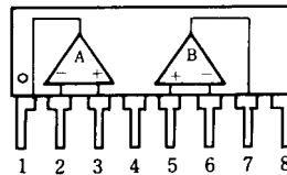
NJM4560L
