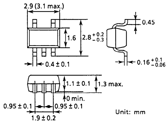
(3) SOT-23-5
